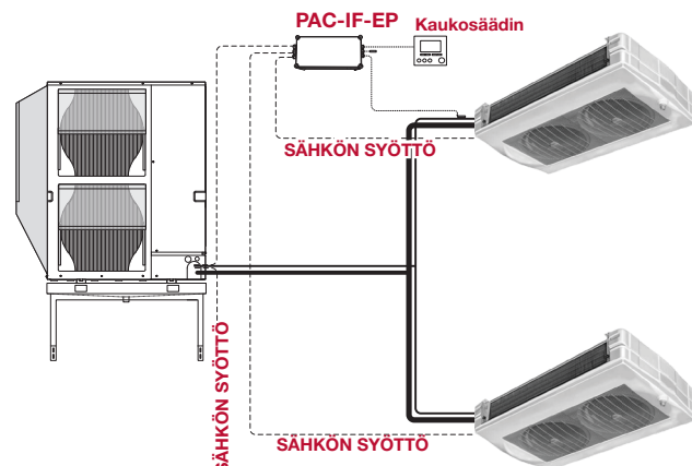
-1 ulkoyksikkö + 2 sisäyksikköä
